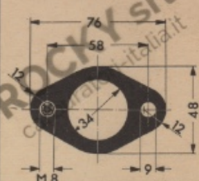
SOLEX-Fallstromvergaser 34 PCI (Hauptschema)
